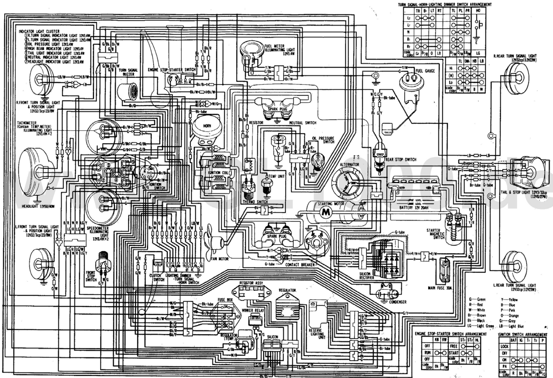
Honda Goldwing GL 1000 – Schaltplan US Modell
